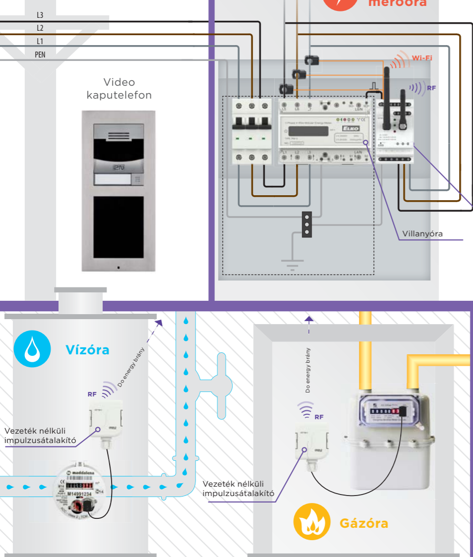
Fogyasztásmérő
